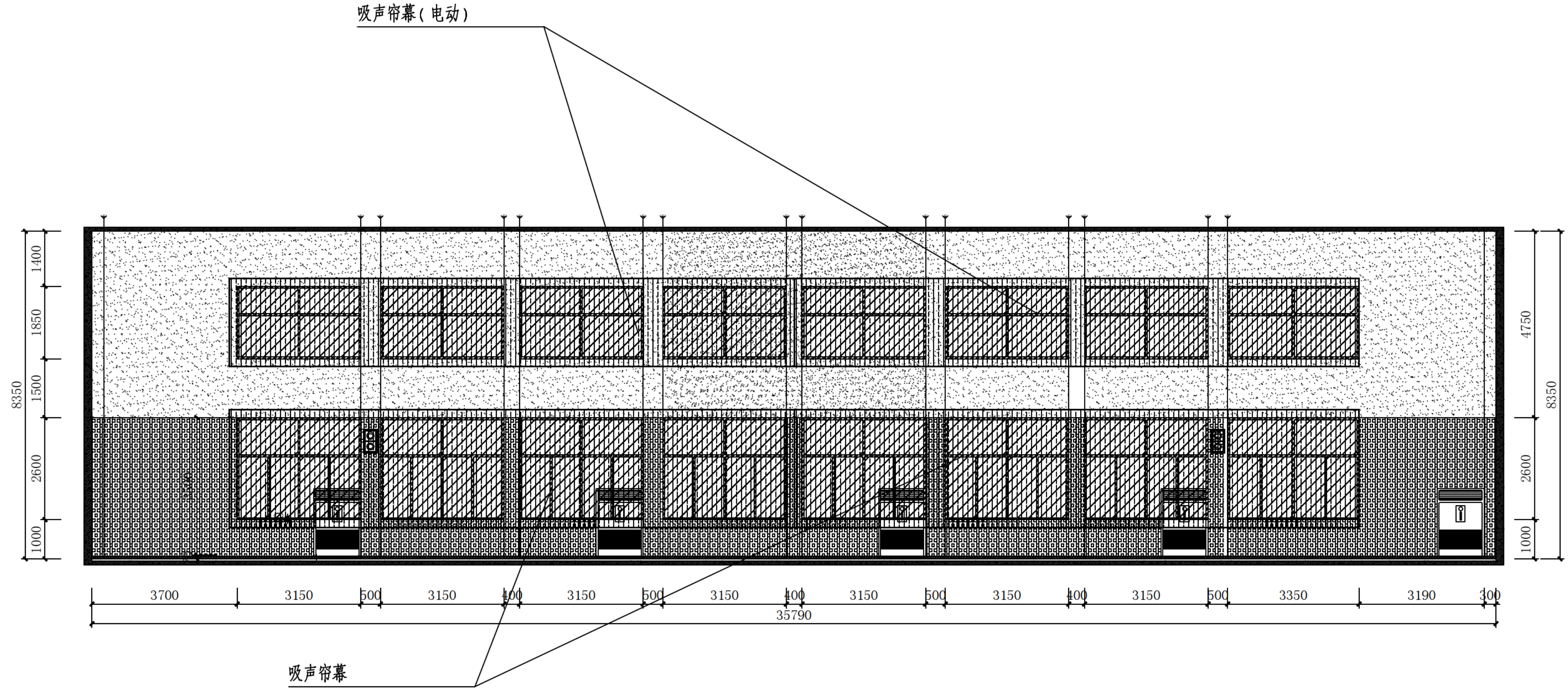
E1 墙面帘幕立面图
