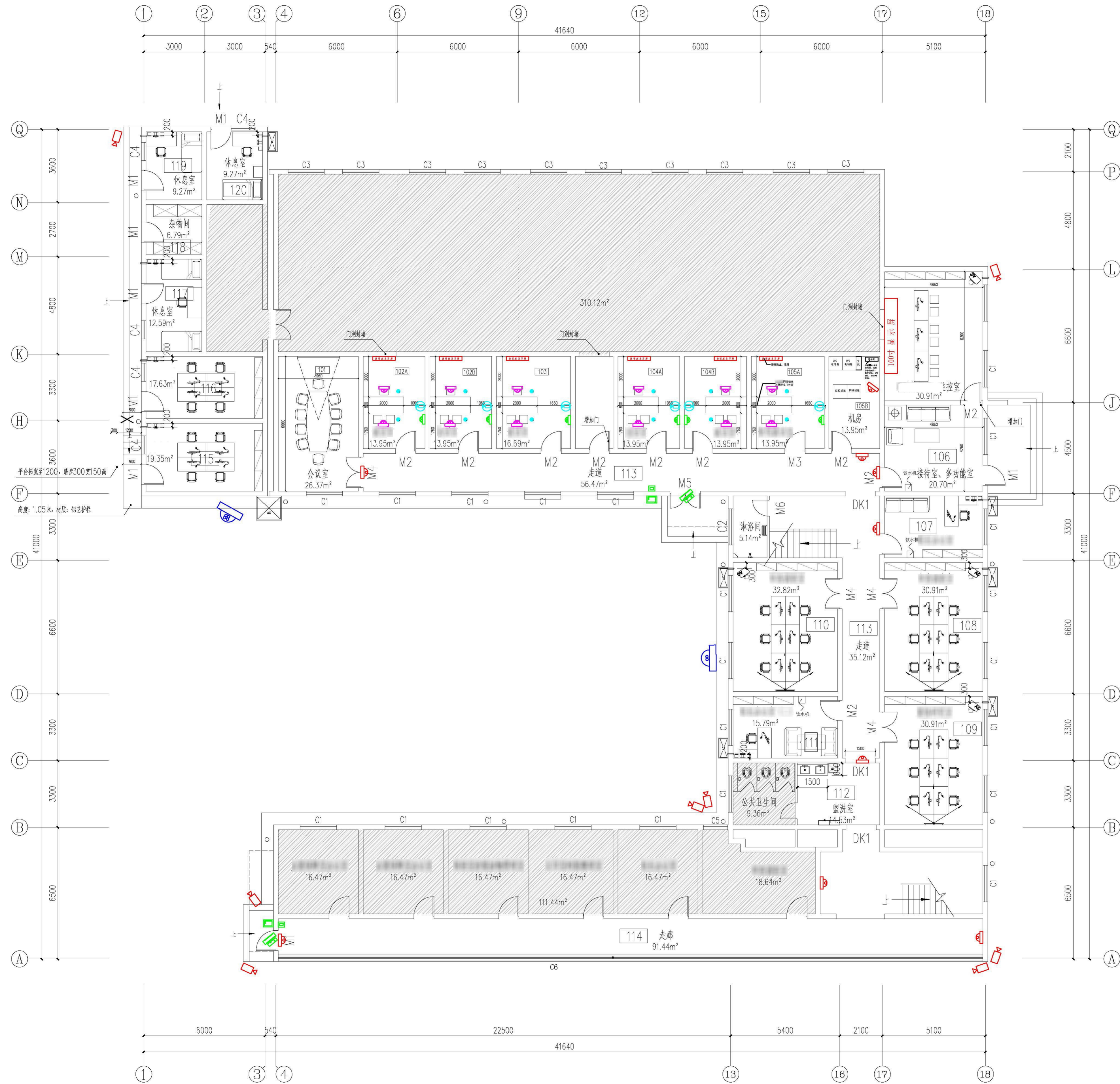
改造一层平面图 1:100
